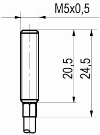
Габаритный чертеж
